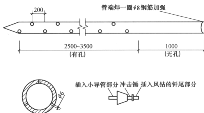
图 4.3.2 小导管结构
